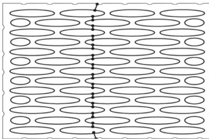
Рисунок А.3 — Приклад найкоротшого шляху між лицьовими гранями для визначення мінімальної суми товщини поздовжніх зовнішніх стінок та внутрішніх перегородок
