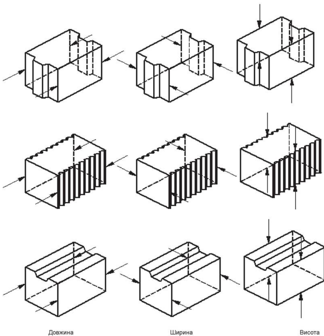
Рисунок 1с) — Позиції вимірювання
