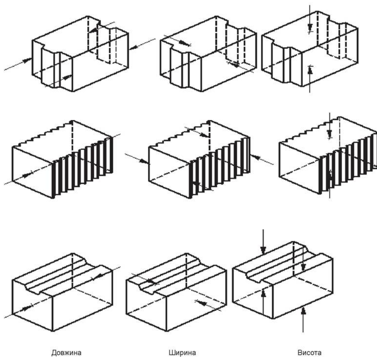
Рисунок 1e) — Позиції вимірювання
