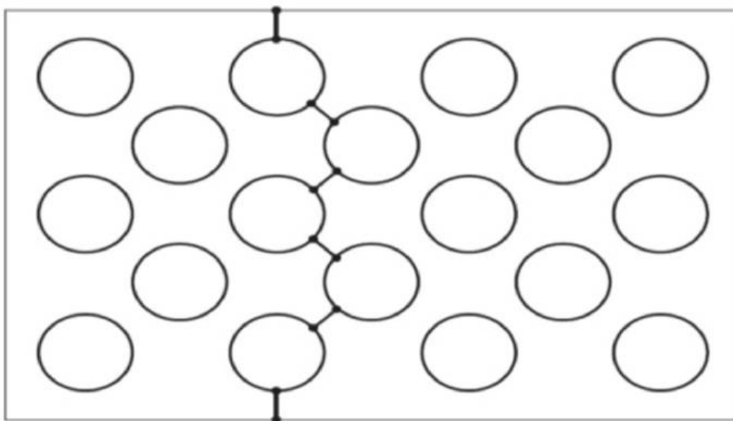
Рисунок А.1 — Приклад найкоротшого шляху між лицьовими гранями для визначення мінімальної суми товщини зовнішніх стінок та внутрішніх перегородок
