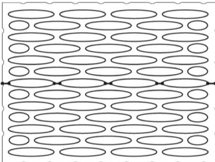
Рисунок А.4 — Приклад найкоротшого шляху від тичка до тичка для визначення мінімальної суми товщини поперечних зовнішніх стінок та внутрішніх перегородок
