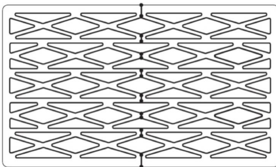
Рисунок А.5 — Приклад найкоротшого шляху між лицьовими гранями для визначення мінімальної суми товщини поздовжніх зовнішніх стінок та внутрішніх перегородок
