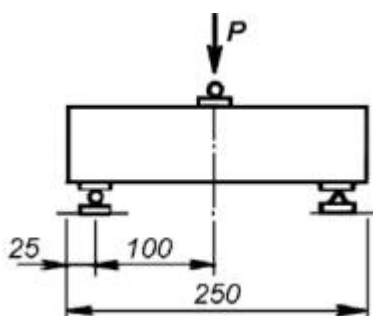
Схема испытания кирпича на изгиб
